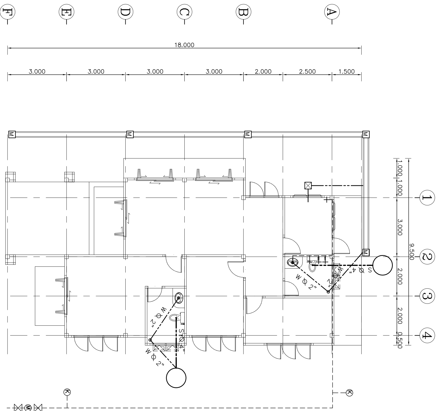
แปลนประปา-สุขาภิบาล SCALE 1:100
